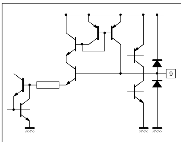
Figure 4 : Pin 9 (YIN)
