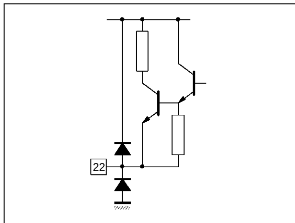
Figure 15 : Pin 22 (DLO)
