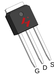
TO-251-3L
